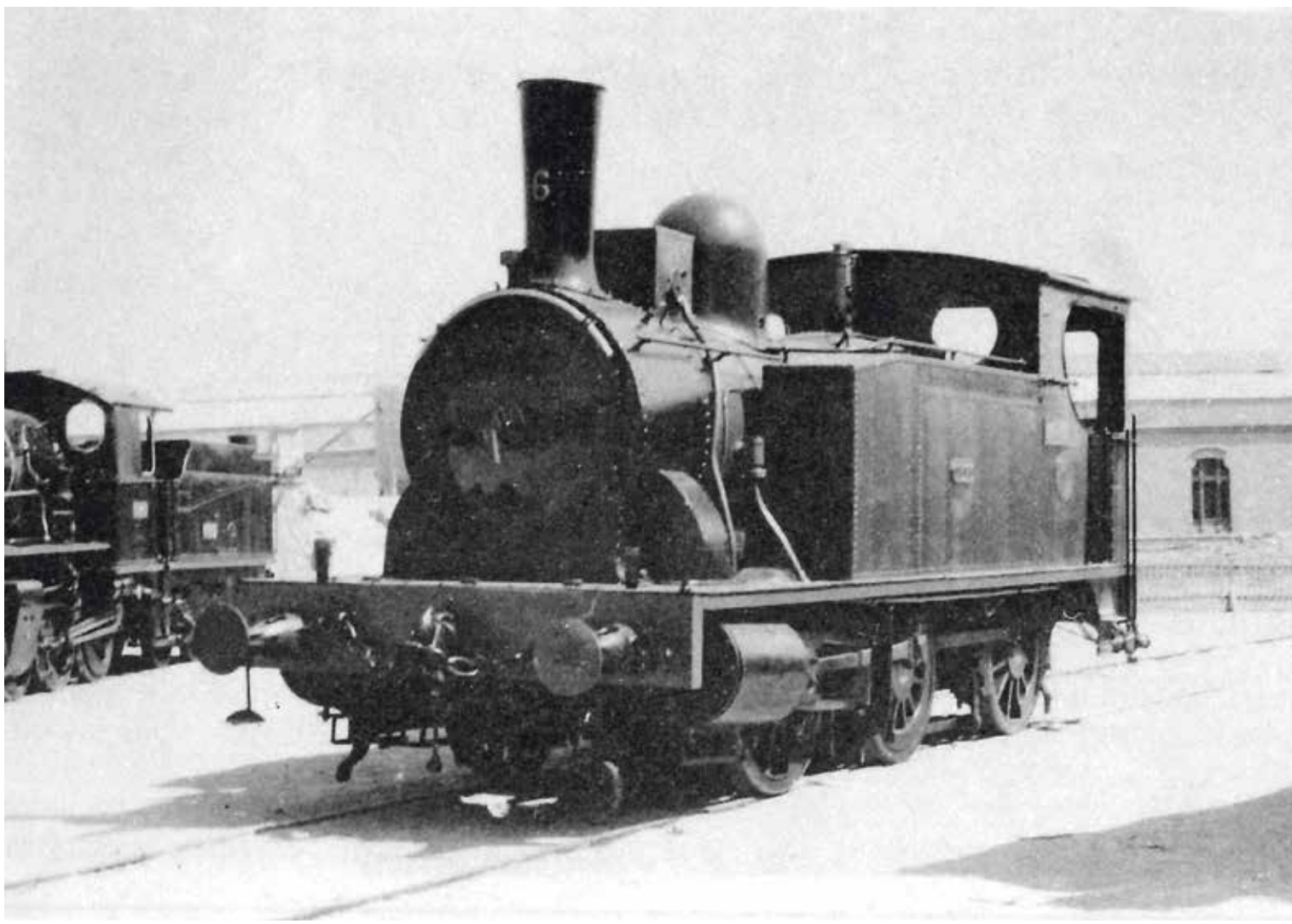
La locomotora Caldes, de 1888, fotografiada al dipòsit de locomotores de la RENFE a Vilanova i la Geltrú. A sota detall de la placa. > AMICS DEL FERROCARRIL
